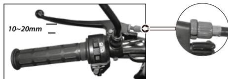
A B Imagen 19. Ajuste de la palanca del embrague.
